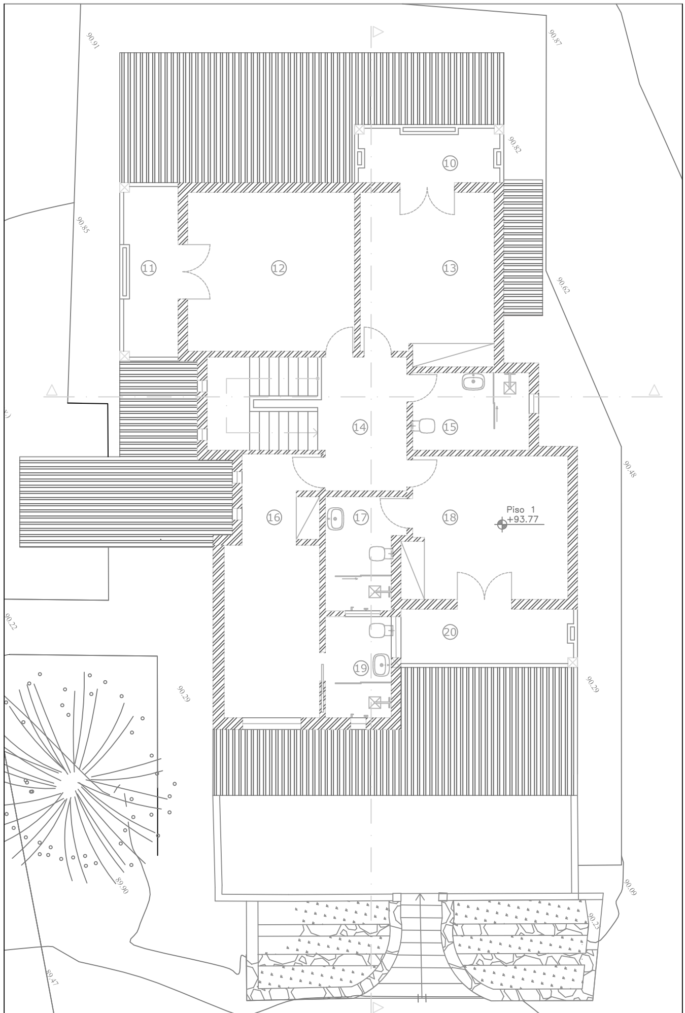
Planta Piso 1 - Proposta
