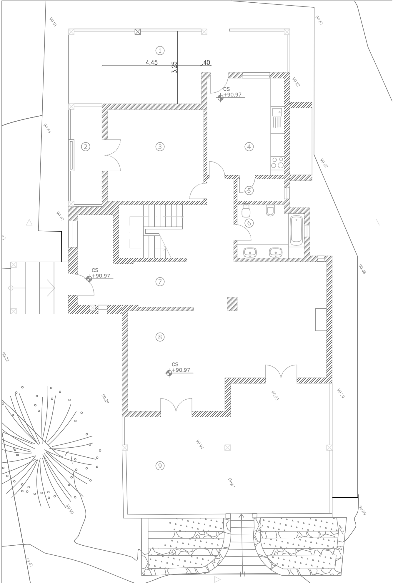
Planta Piso 0 - Proposta
