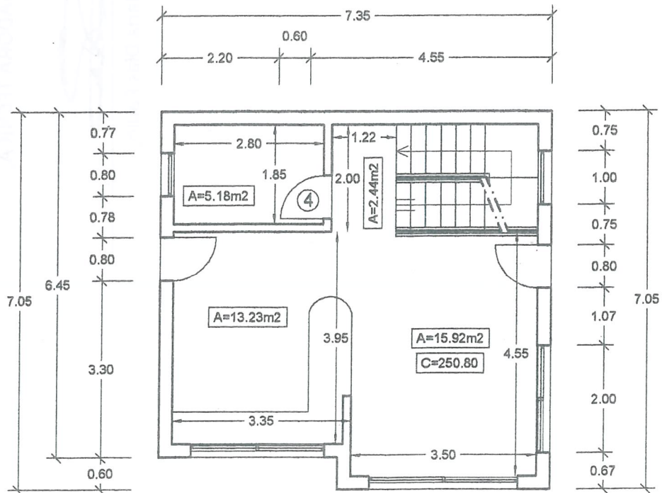
PLANTA DA CAVE
