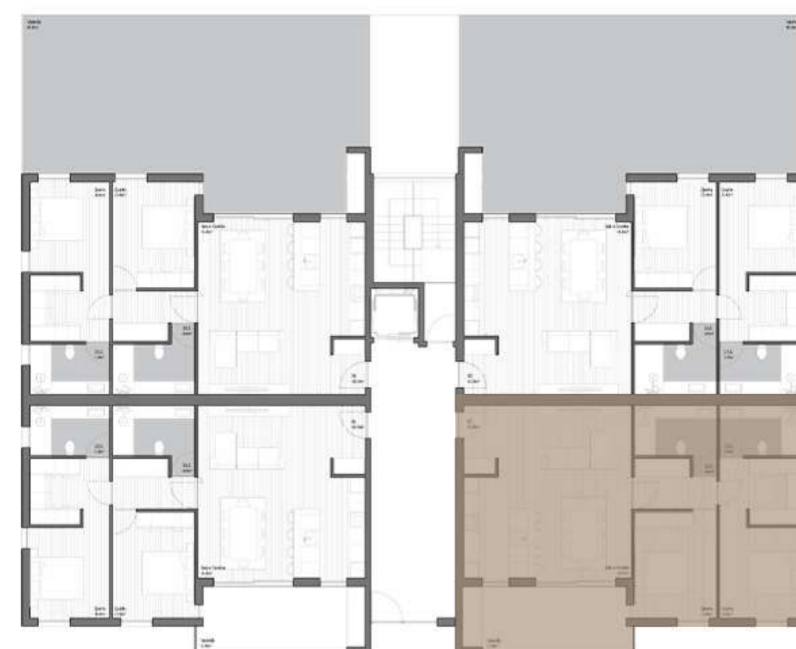
FRAÇÃO 0C
