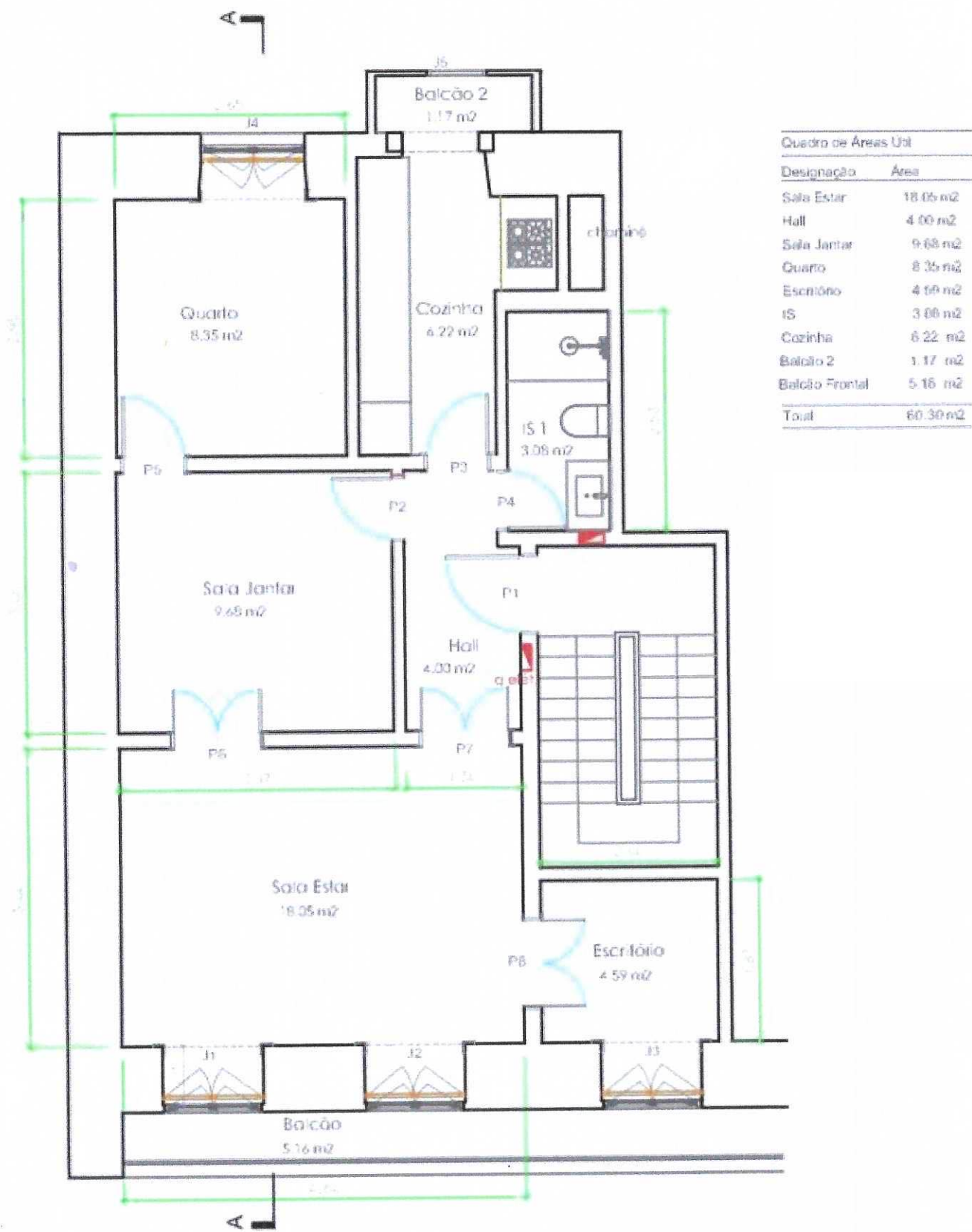
Manuel Bernardes 214 E Planta escala: 1:100
