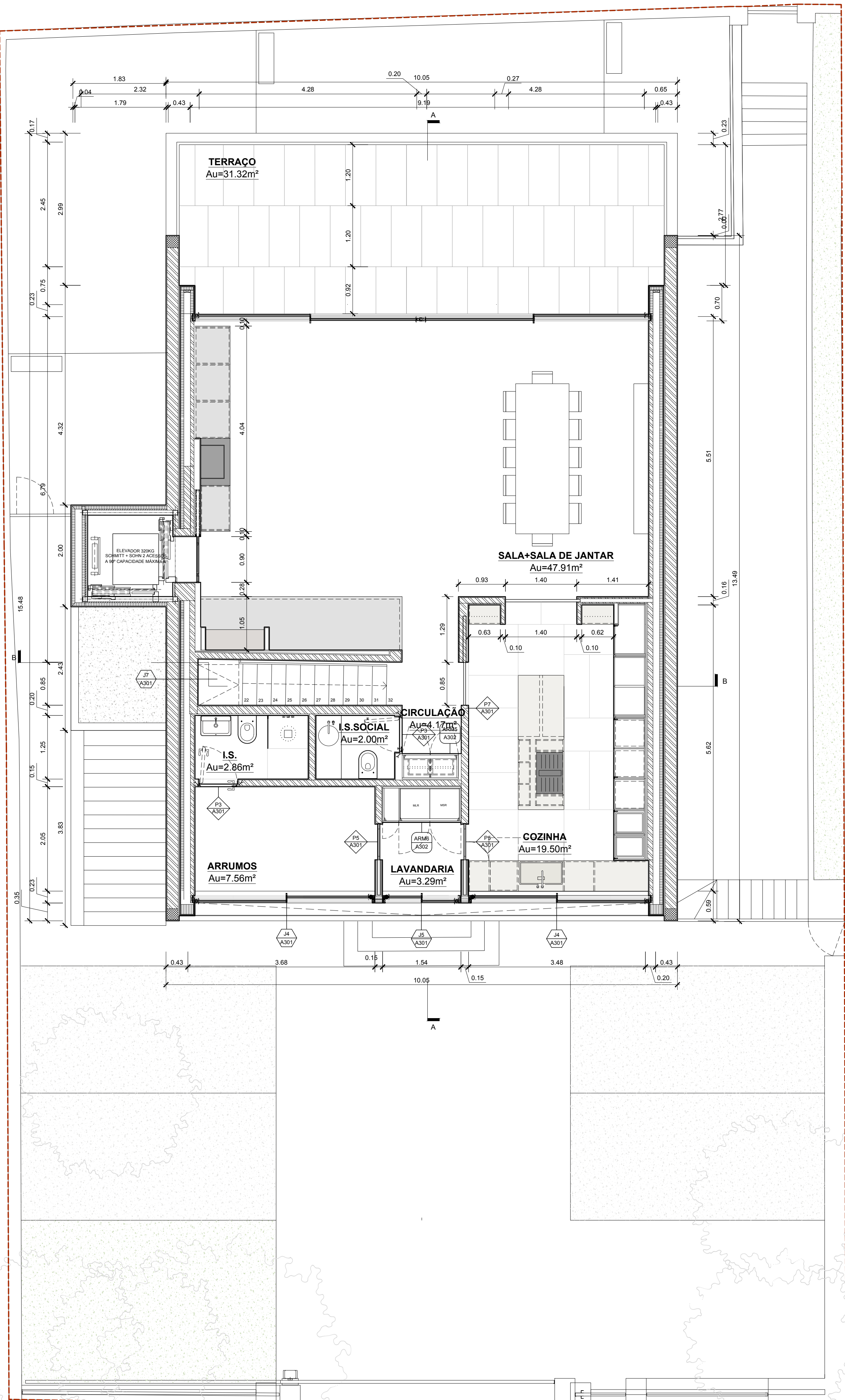
2 PLANTA SOTÃO - PROPOSTA escala 1:50
