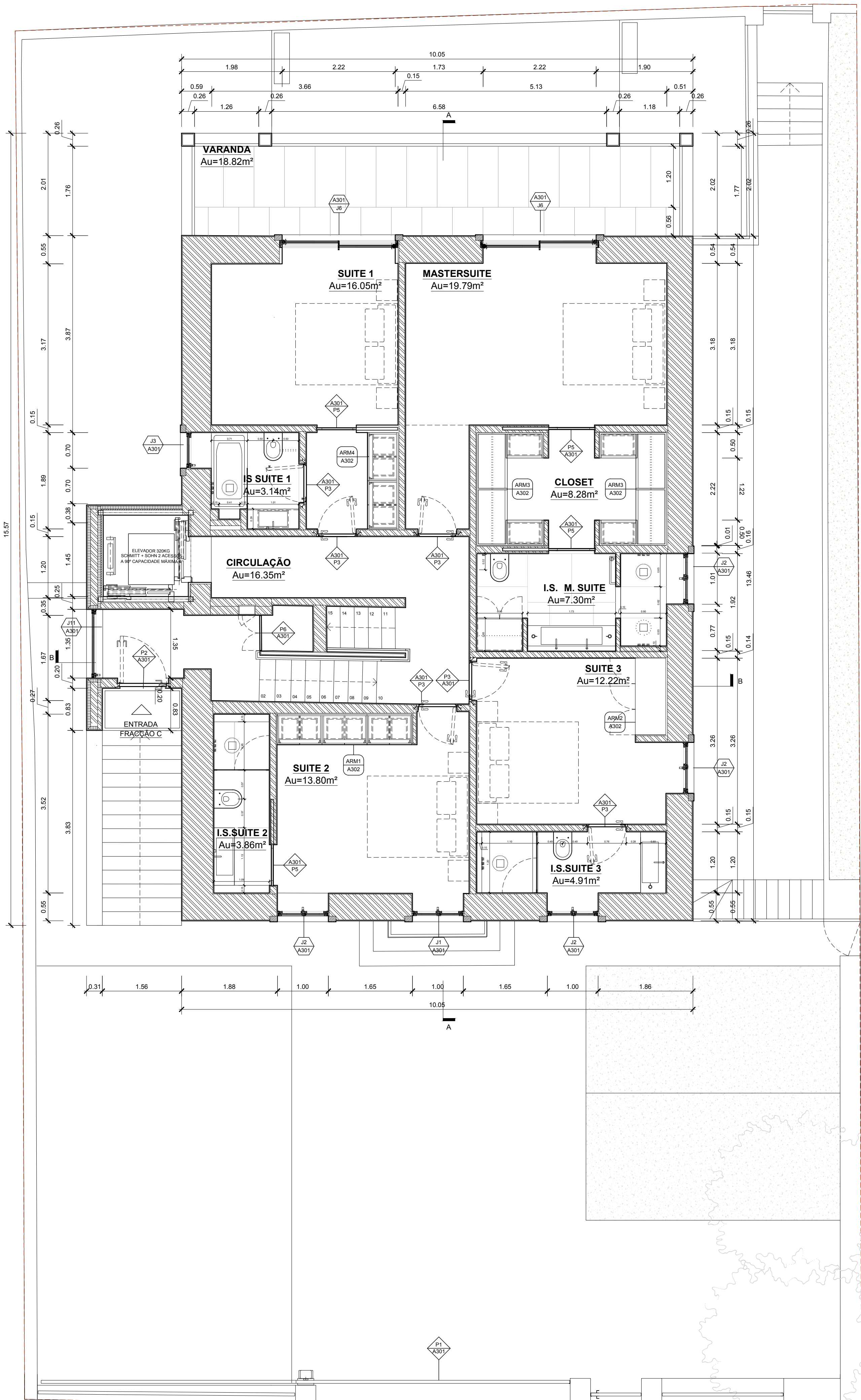
1 PLANTA 1º ANDAR - PROPOSTA escala 1:50
