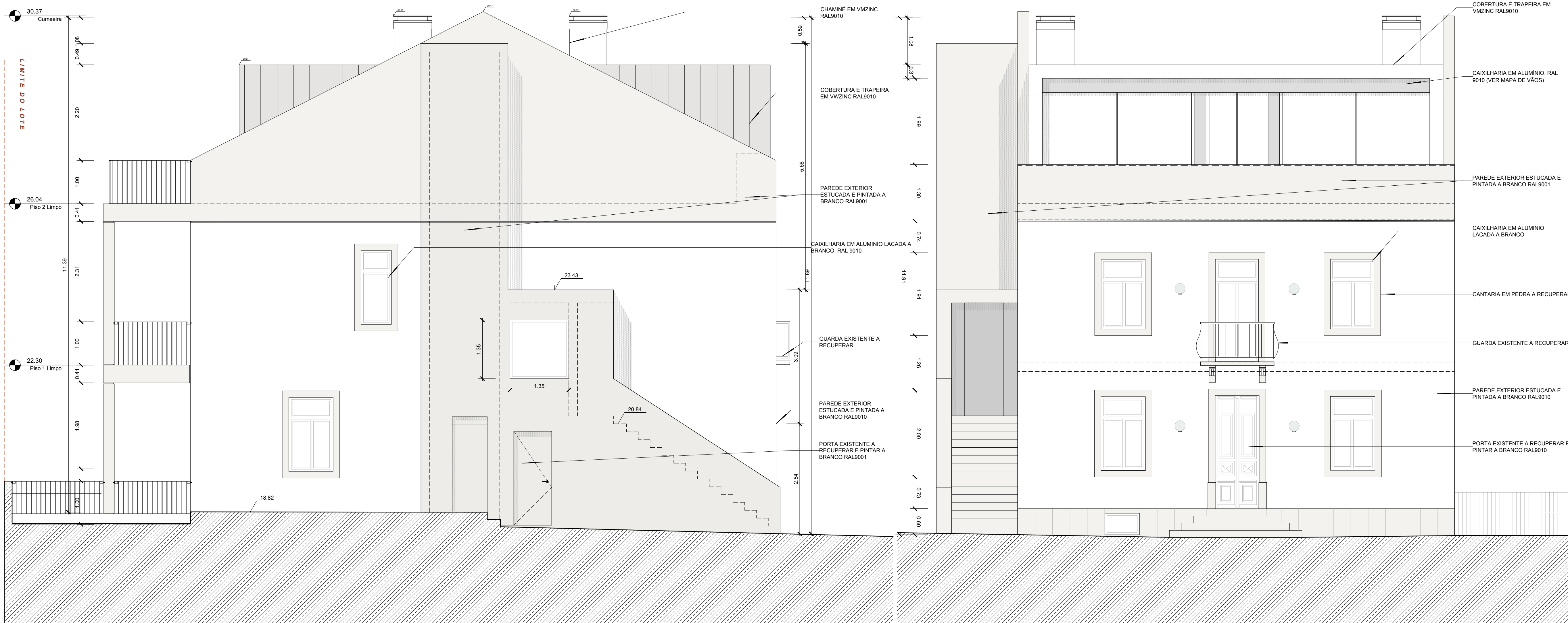
4 ALÇADO ESTE - PROPOSTA escala 1:50
