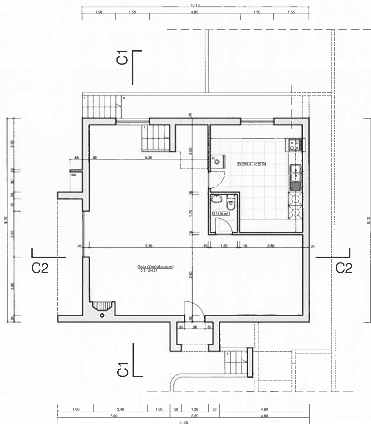
PLANTA DO PISO 0 PROPOSTO
