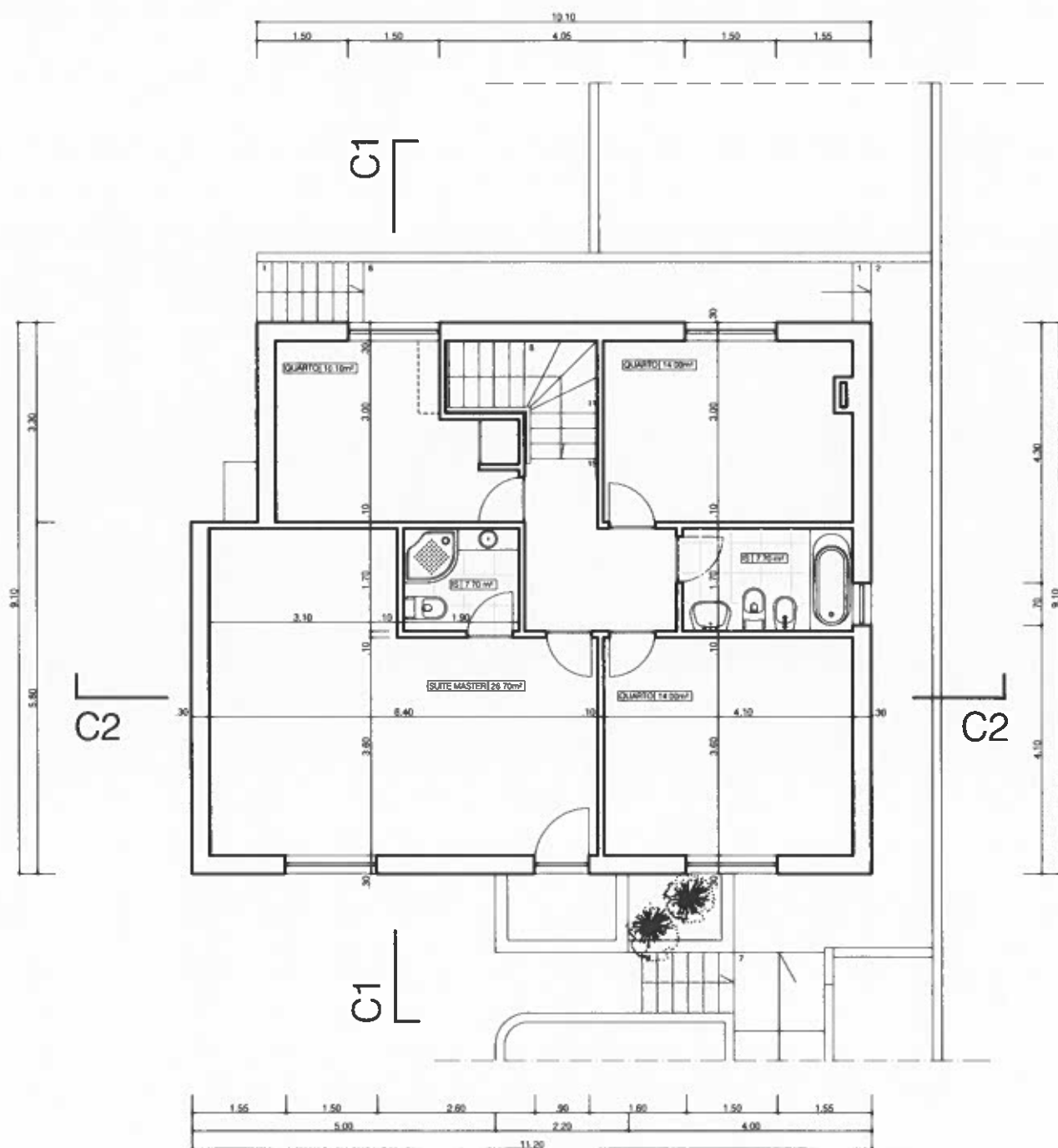
PLANTA DO PISO 1 PROPOSTO
