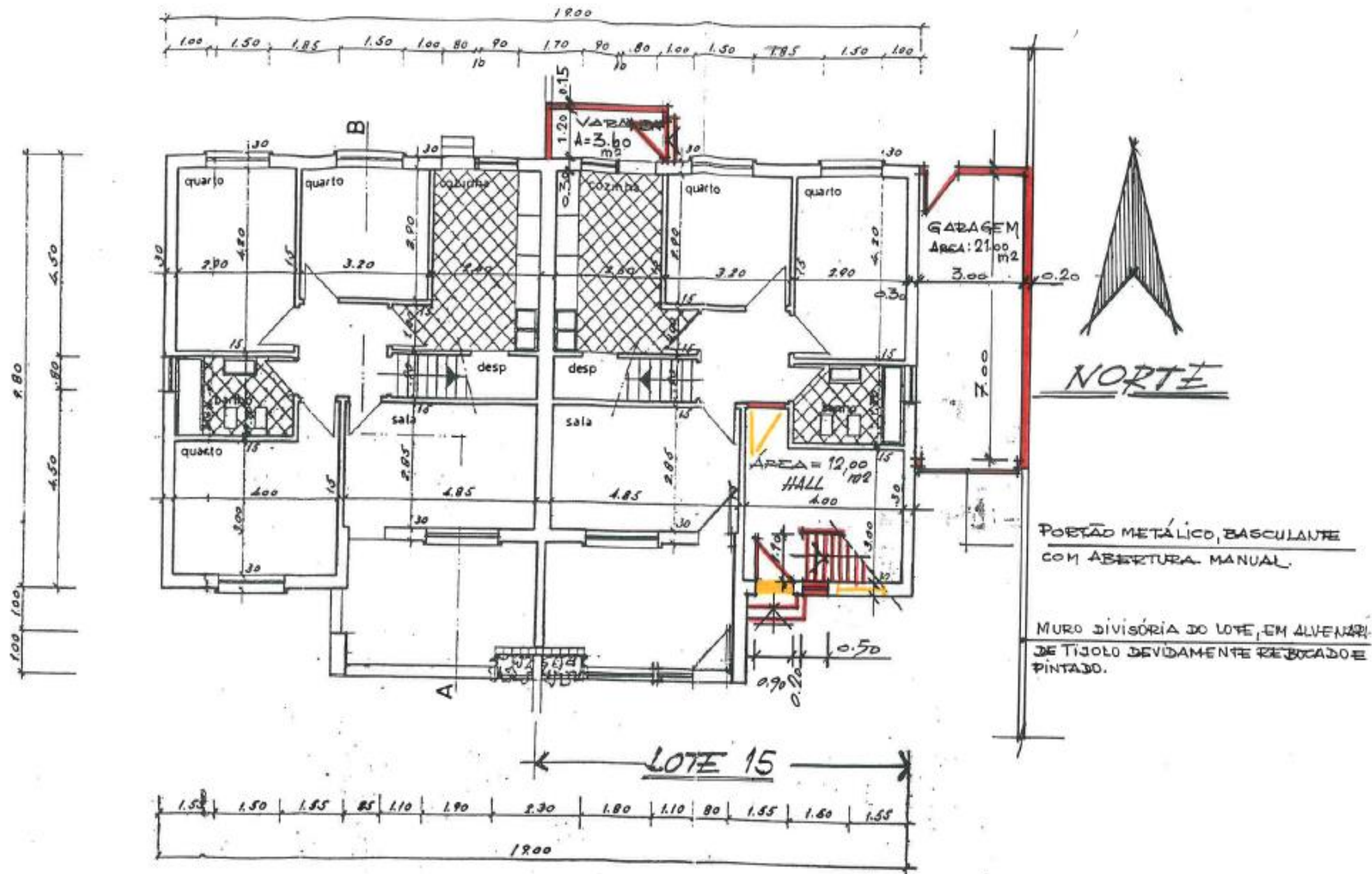
PLANTA DO R/C
