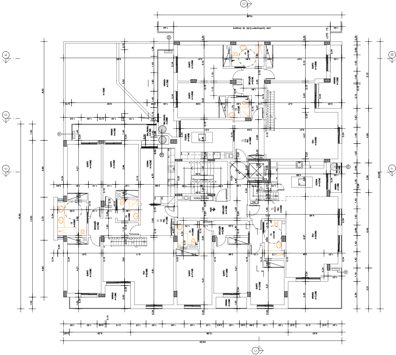
PLANTA PISO 4 ÁREA DO PISO = 441,57m 2 ÁREA VAREJOS = 55,582
