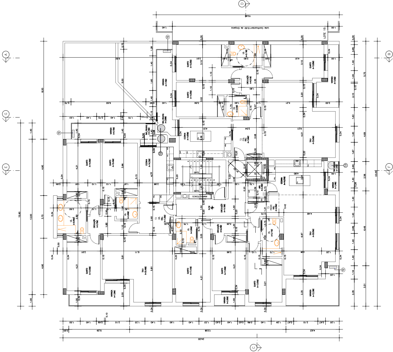
PLANTA PISO 3 ÁREA DO PISO = 441,57m 2 ÁREA VÍDEOS = 55,582
