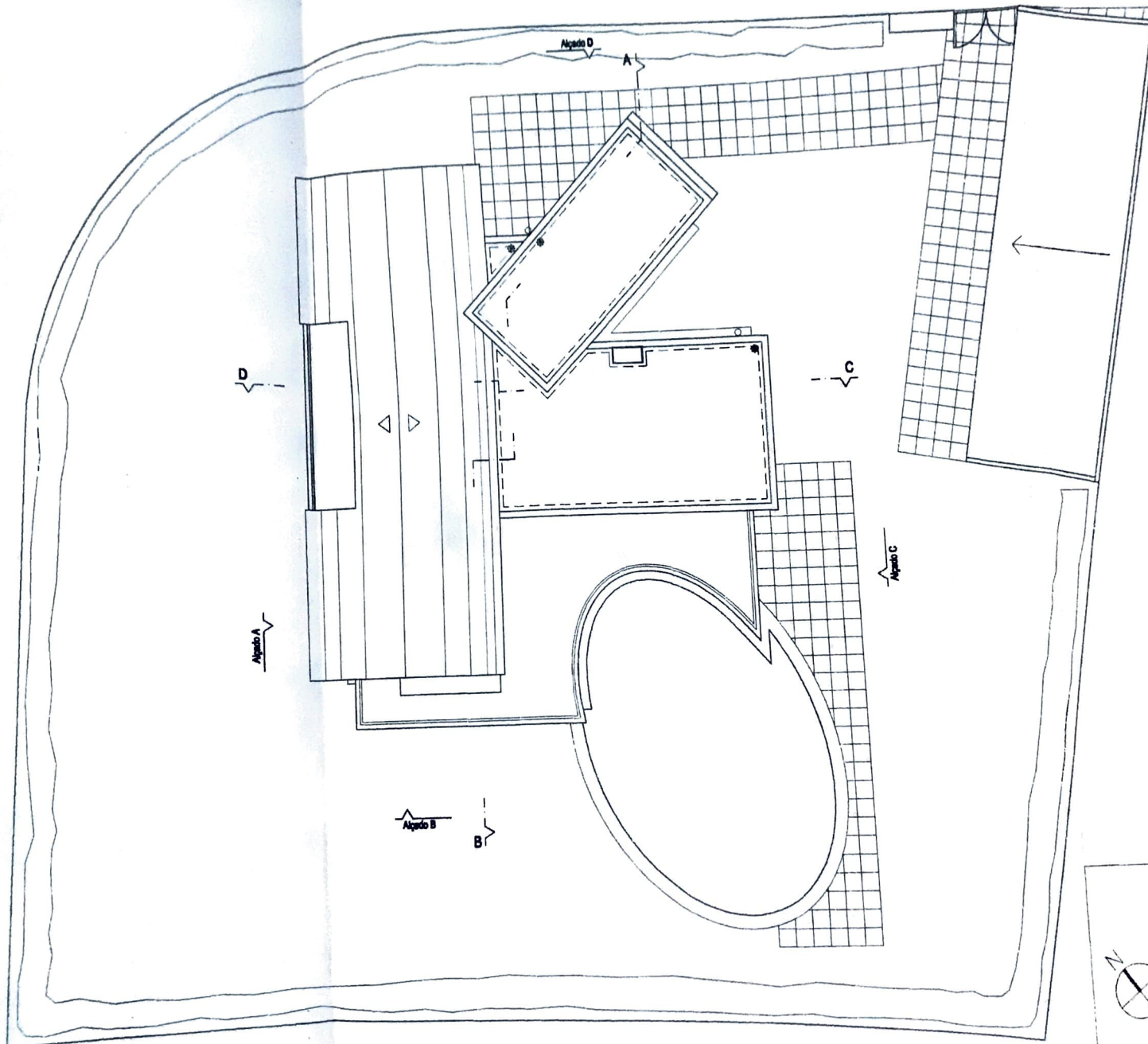
PLANTA DE COBERTURAS
