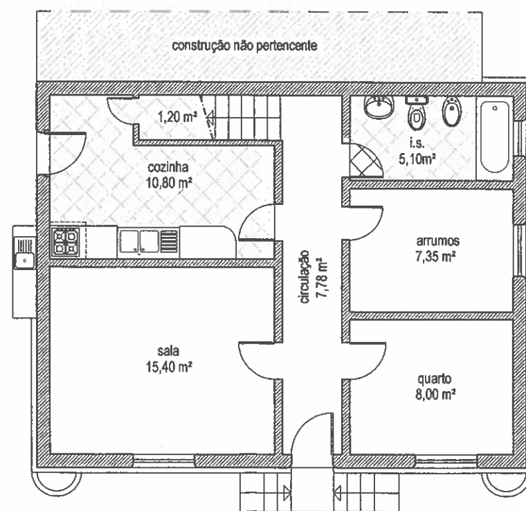
PISO TÉRREO
