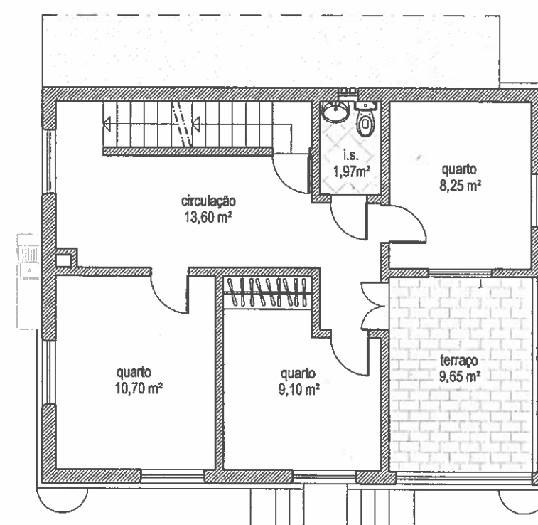
PISO SUPERIOR
