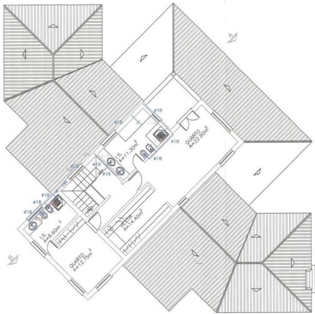
PLANTA DO PISO 1 A=72.00 m 2
