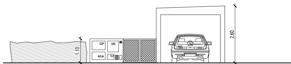
ALÇADO FRONTAL
