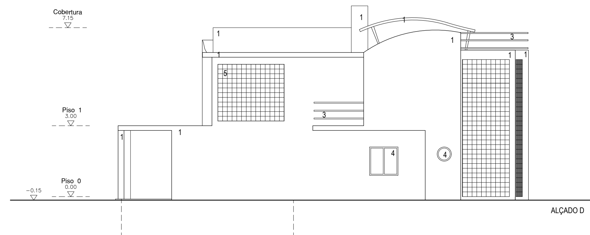
ALÇADO C
