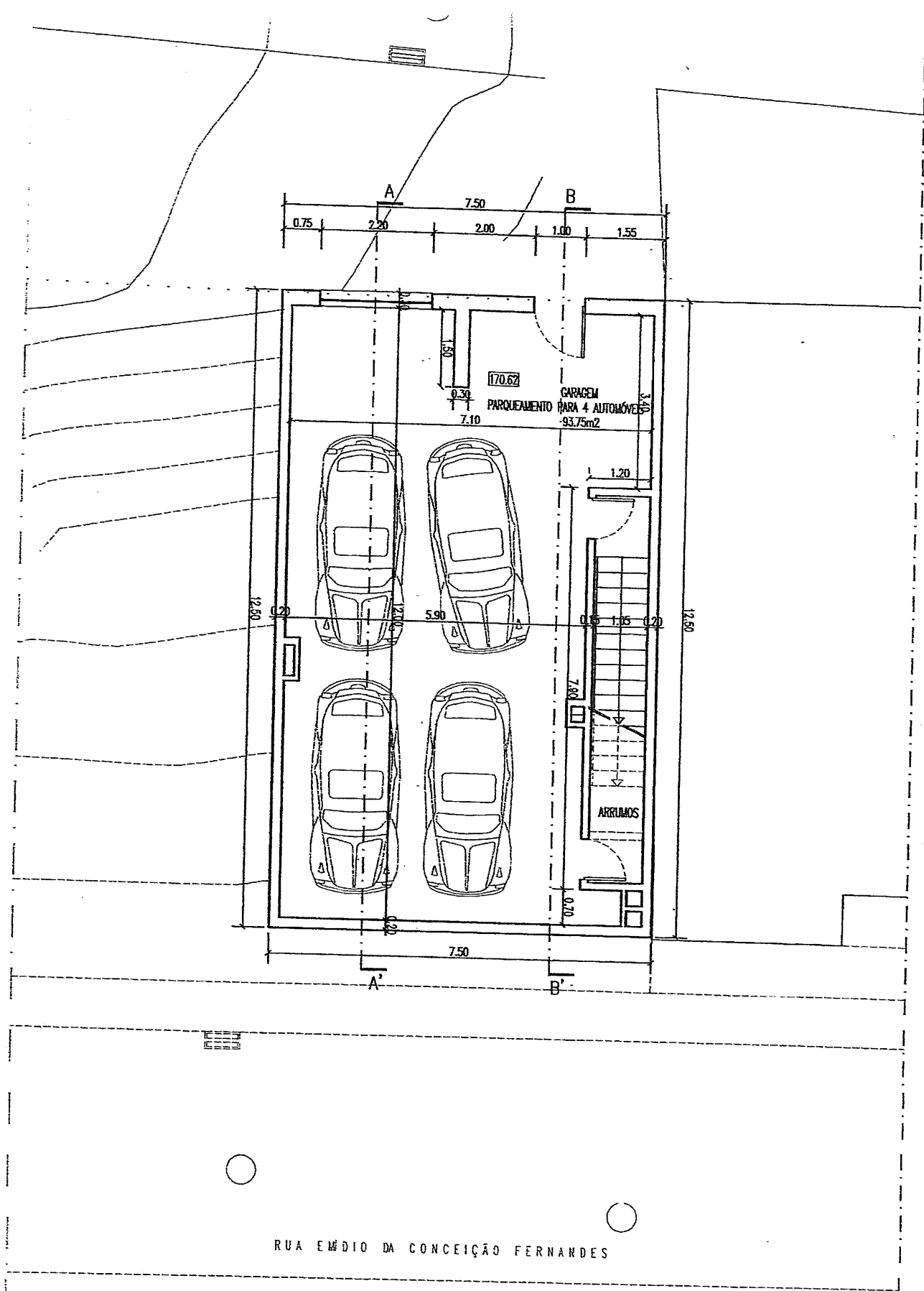
PLANTA DA CAVE
