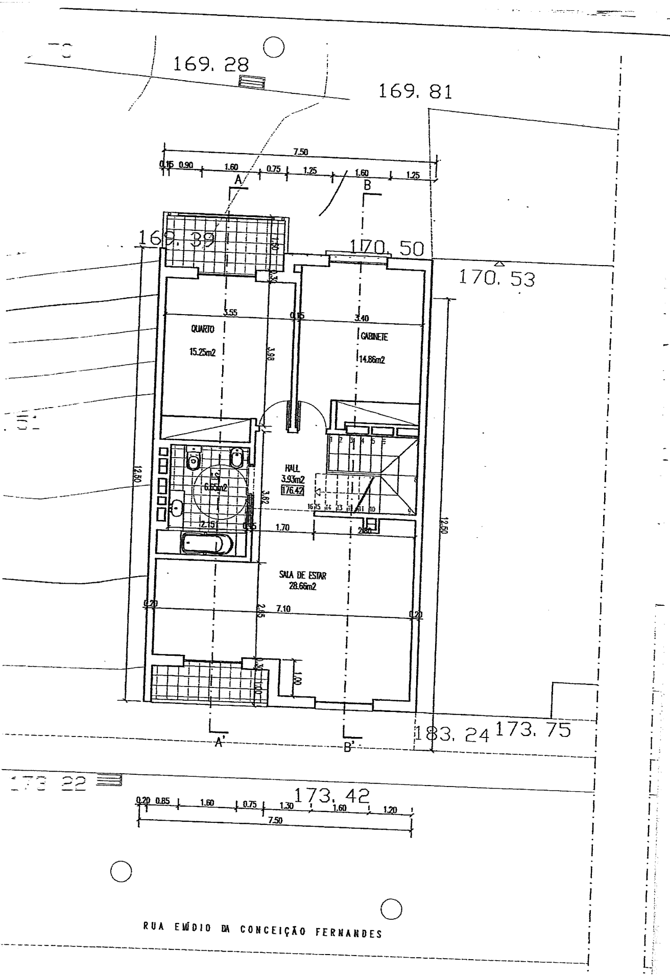
PLANTA DO 1º PISO
