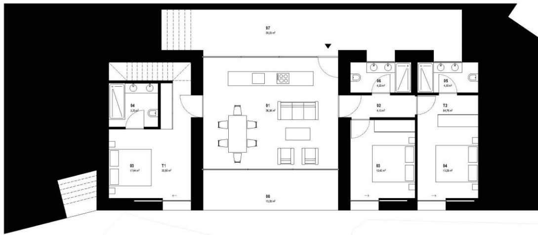
Piso 0
