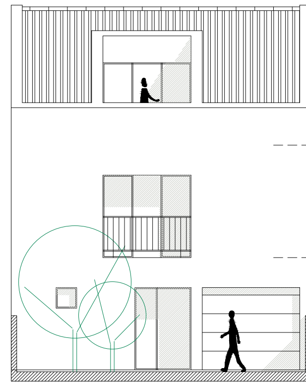
ALÇADO PRINCIPAL
