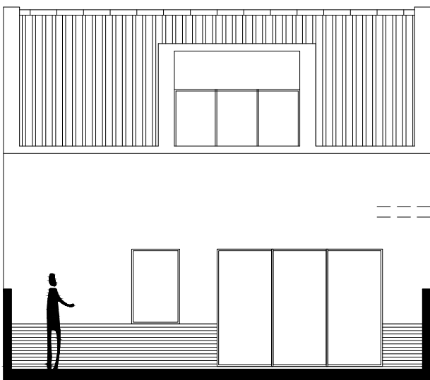
ALÇADO TARDOZ
