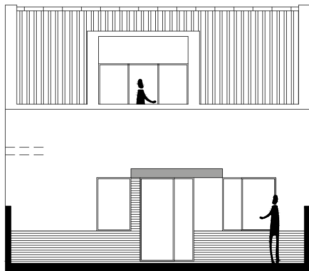
ALÇADO PRINCIPAL
