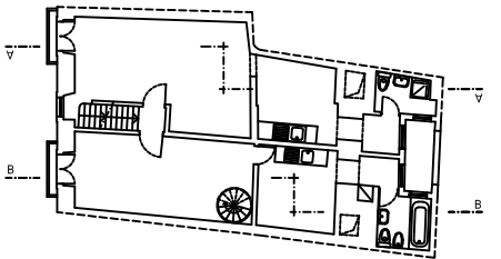
PLANTA DO PISO 4
