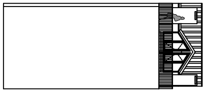
ALÇADO TABEZO
