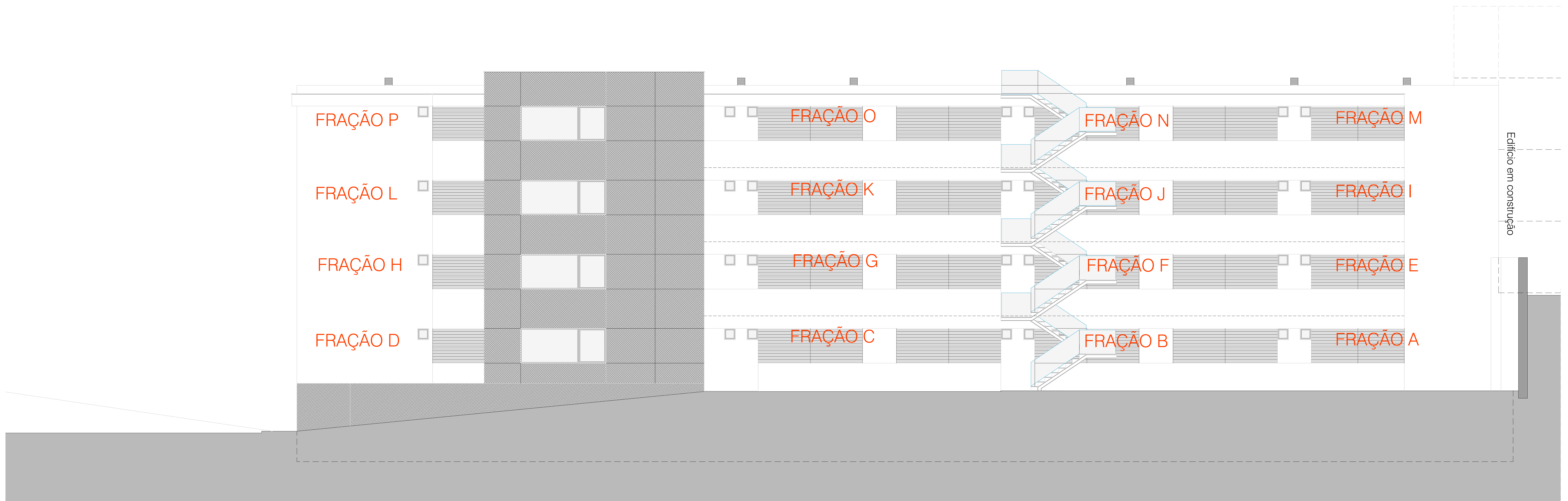
ALÇADO - NORTE
