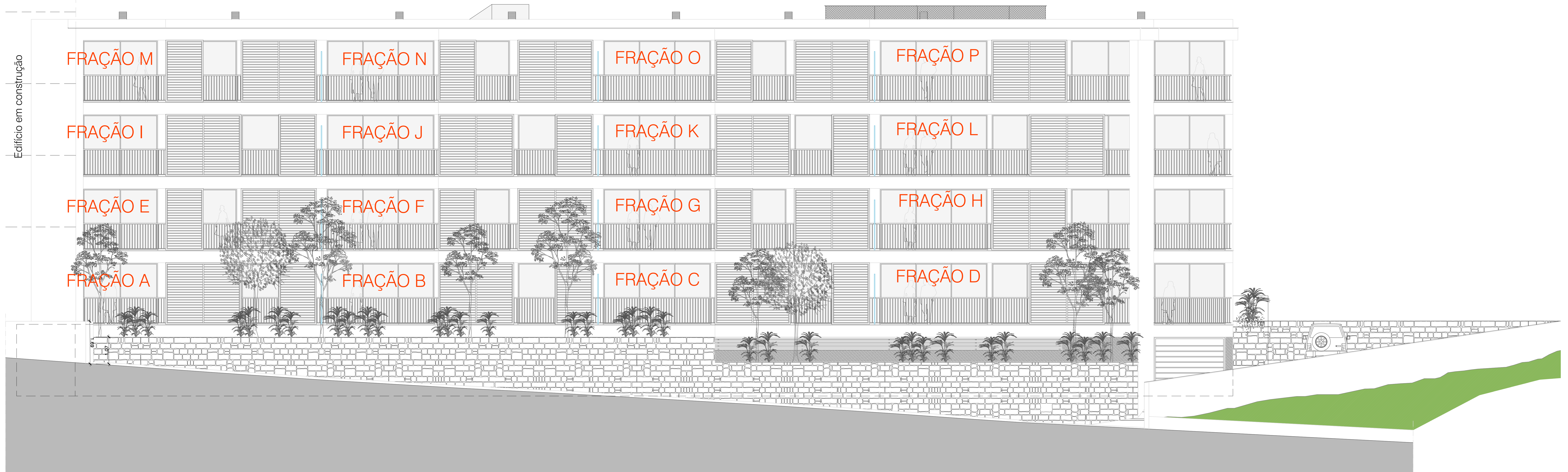
ALÇADO - SUL
